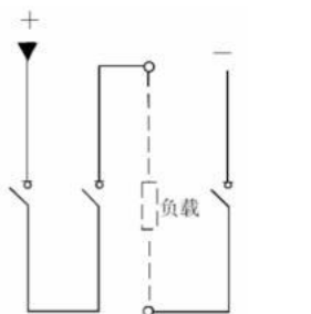
3P外形接线图(DC500V)
